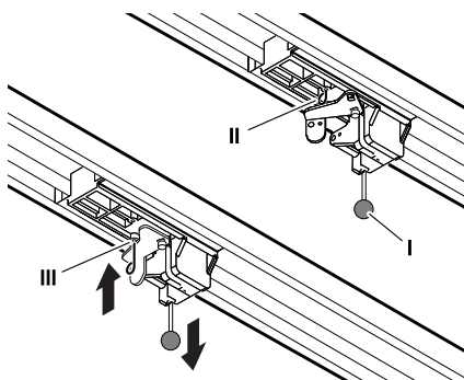
III. 16: Låse og låse opp drev
