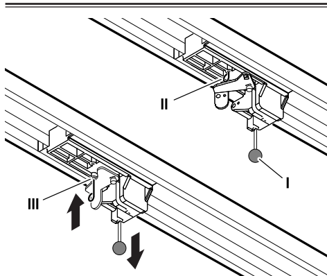
Obr. 16: Odblokování a zablokování pohonu
