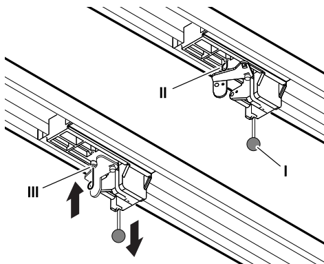
Obr. 6: Odblokování a zablokování pohonu
