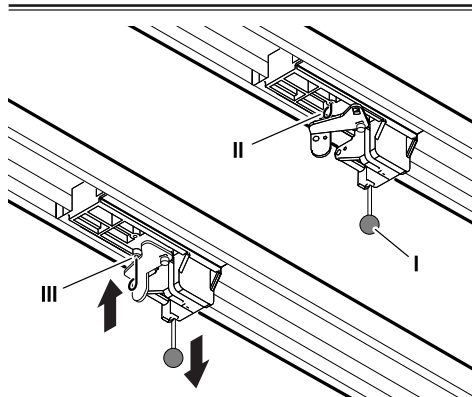
Fig. 16: Låsa upp och låsa drivenheten
