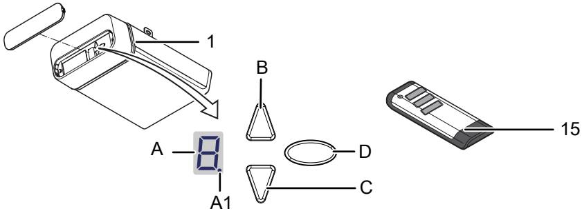
Kuva 2: Hallintalaitteet
