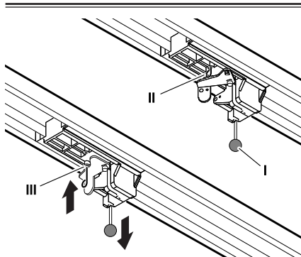
Kuva 16: Avaajan kytkeminen irti ja lukitseminen
